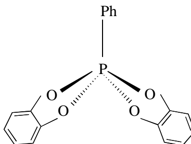
Phenylbis(1,2-benzenedioxy)phosphorane
