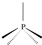
TetragonalPyramid (TP)
